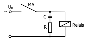
Unterdrückung von Spannungsspitzen mit einem RC-Glied
