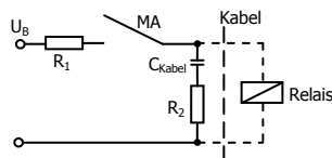
Kontaktschutz mit Widerständen zur Strombegrenzung
