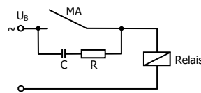
Unterdrückung von Spannungsspitzen mit einem RC-Glied
