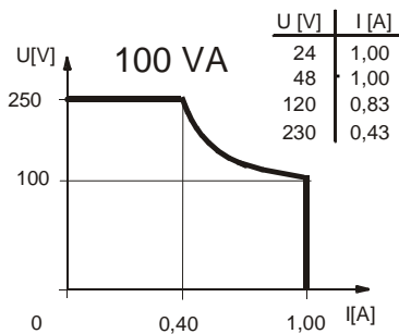
Leistungsdiagramm
