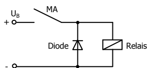
Unterdrückung von Spannungsspitzen mit einer Freilaufdiode
