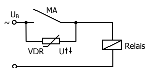
Unterdrückung von Spannungsspitzen mit einem VDR
