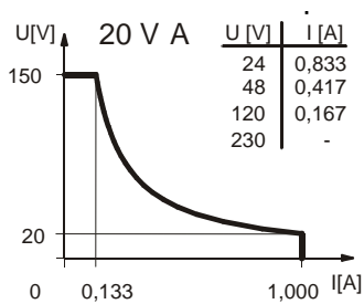
Leistungsdiagramm
