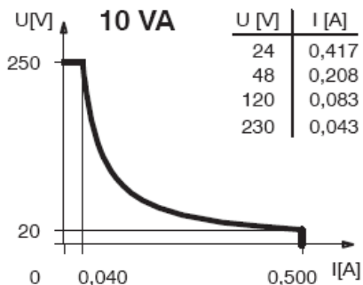
Leistungsdiagramm
