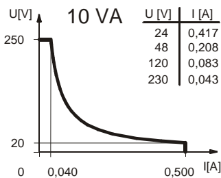
Leistungsdiagramm
