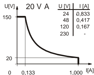
Leistungsdiagramm
