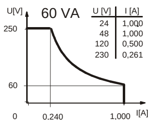
Leistungsdiagramm
