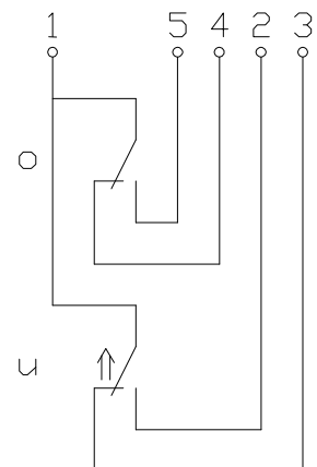
Anschlußschema (ohne Flüssigkeit)
