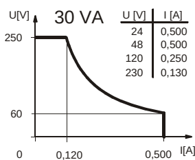
Leistungsdiagramm
