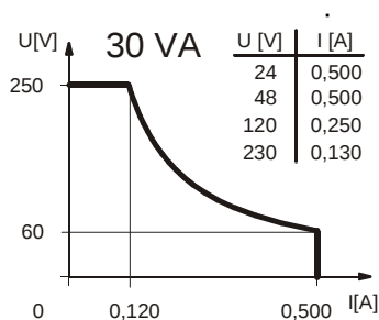
Leistungsdiagramm
