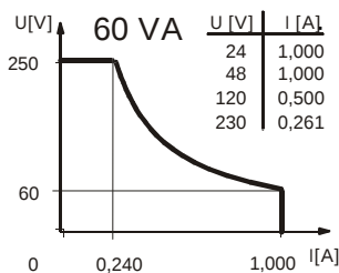
Leistungsdiagramm
