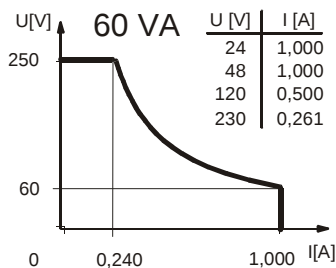
Leistungsdiagramm
