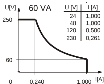
Leistungsdiagramm
