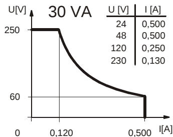
Leistungsdiagramm
