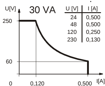
Leistungsdiagramm
