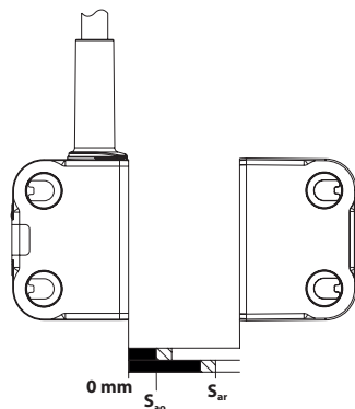
Anfahrriechung / Schaltabstand
