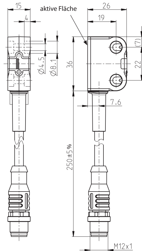
Maßbild
