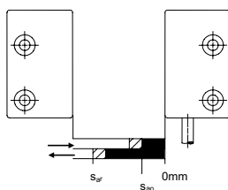
Anfahrriechung / Schaltabstand
