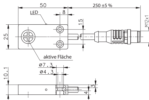
Maßbild
