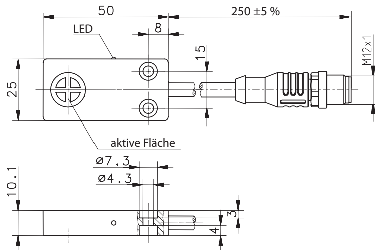
Maßbild
