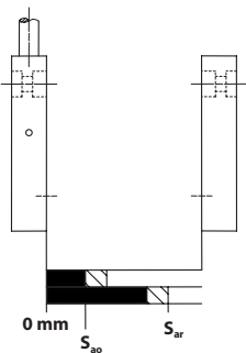
Anfahrriktung / Schaltabstand
