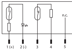
Anschlussbild
