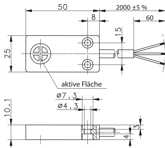
Maßbild
