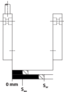
Anfahrrichtung / Schaltabstand
