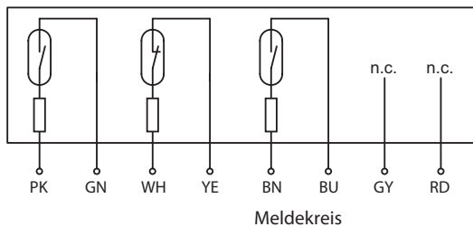
Anschlussbild
