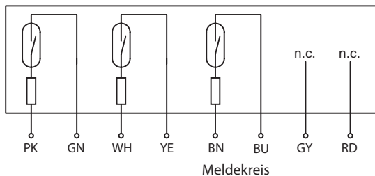
Anschlussbild
