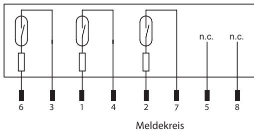
Anschlussbild
