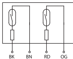
Anschlussbild
