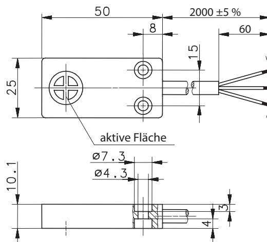
Maßbild
