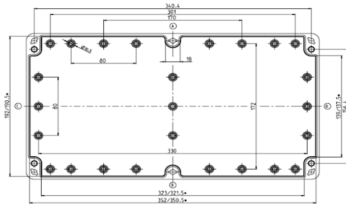
Unterteil
