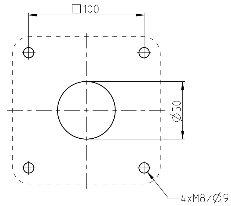
Bearbeitungszeichnung für Montagefläche
