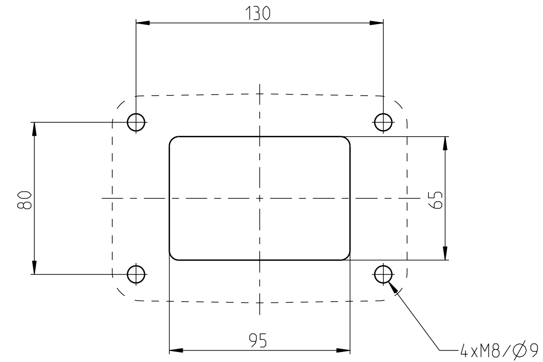
Bearbeitungszeichnung für Montagefläche
