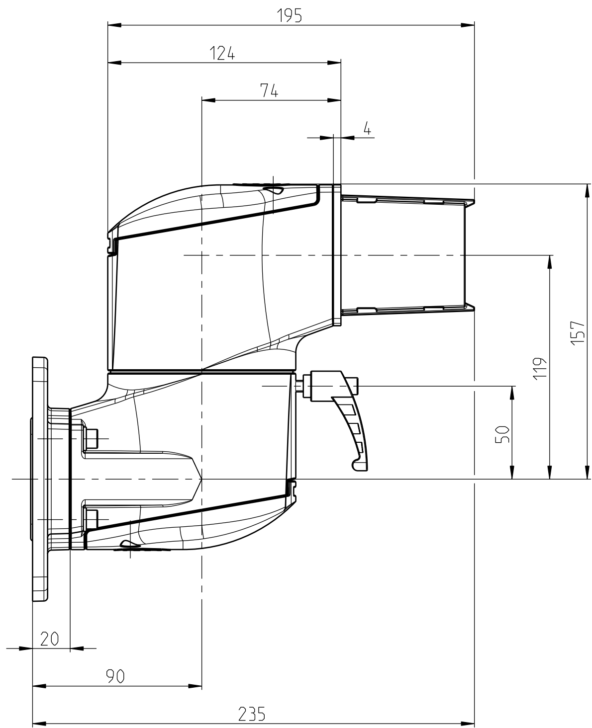
Bearbeitungszeichnung für Montagefläche
