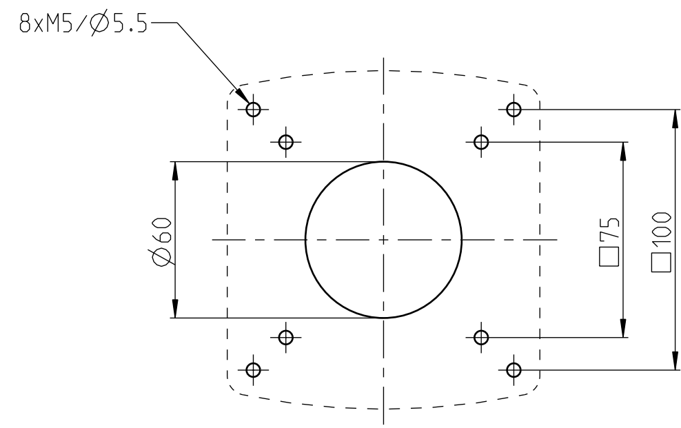
Bearbeitungszeichnung für Montagefläche
