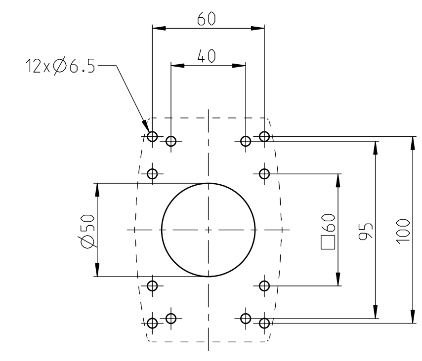
Bearbeitungszeichnung für Montagefläche
