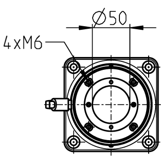
CS-3000 Standfußkupplung Art.-Nr. 1015300183
