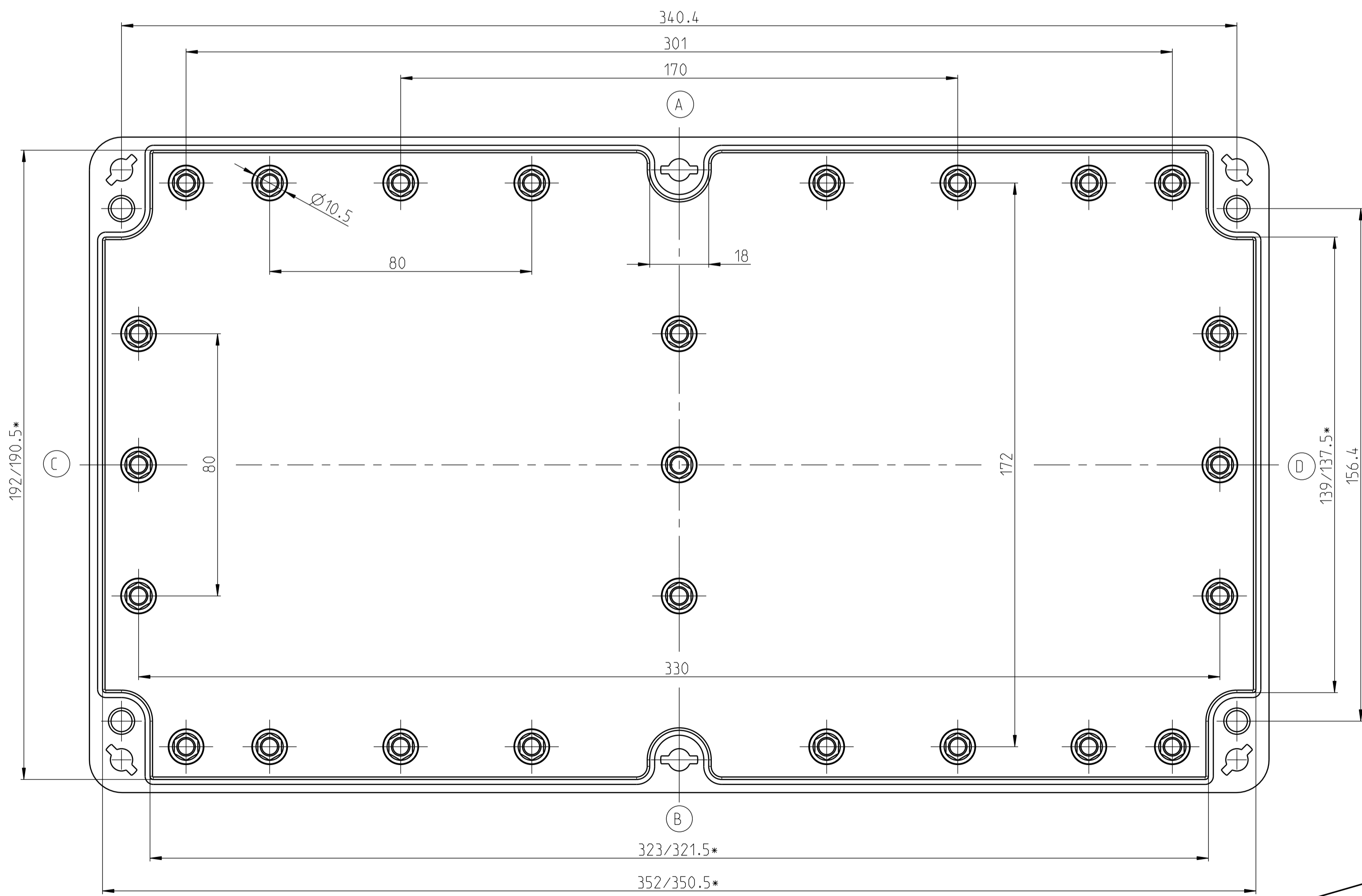
UNTERTEIL/BASE/PARTIE BASSE
