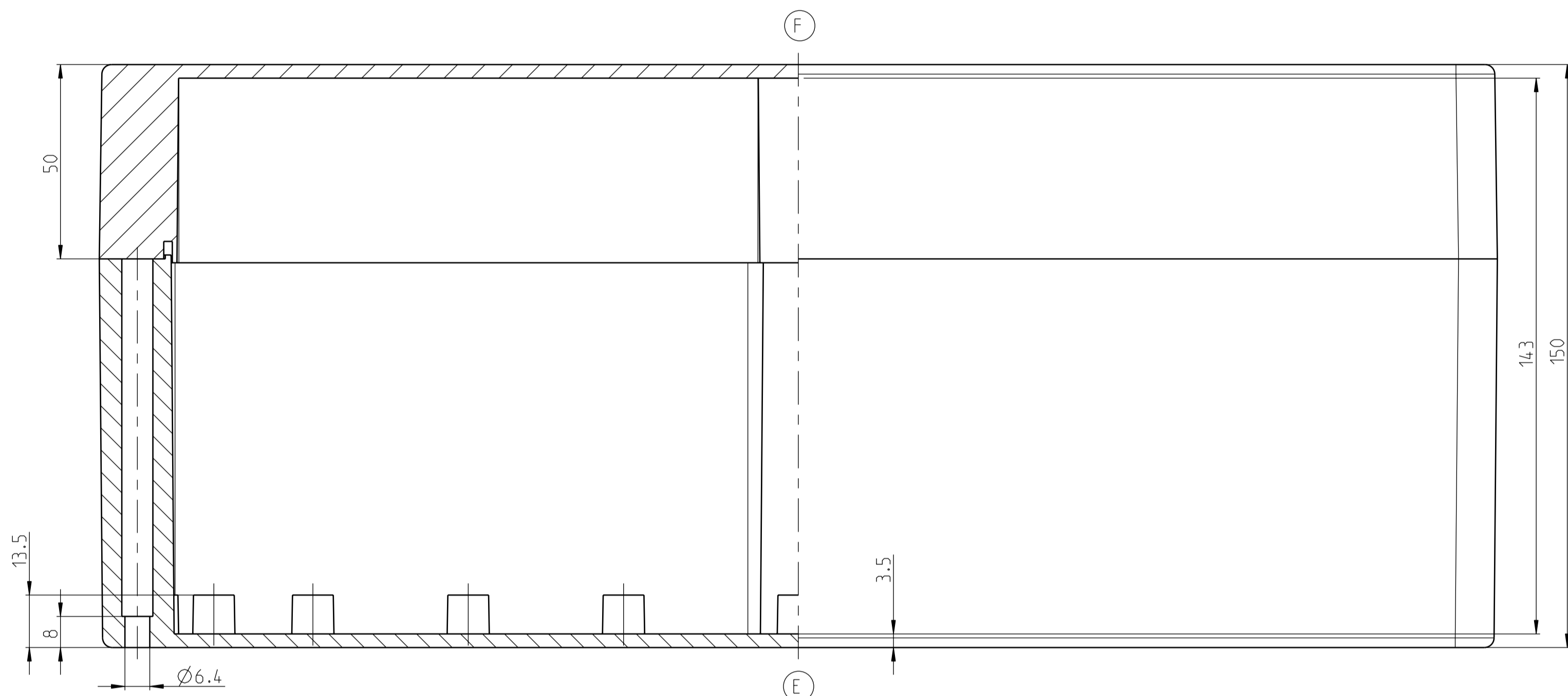
UNTERTEIL/BASE/PARTIE BASSE
