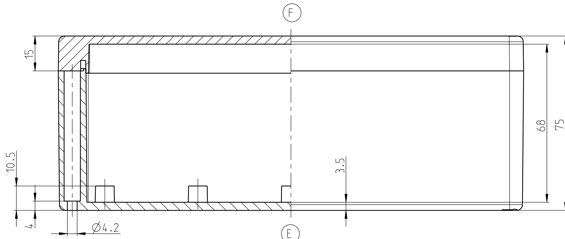
UNTERTEIL/BASE/PARTIE BASSE
