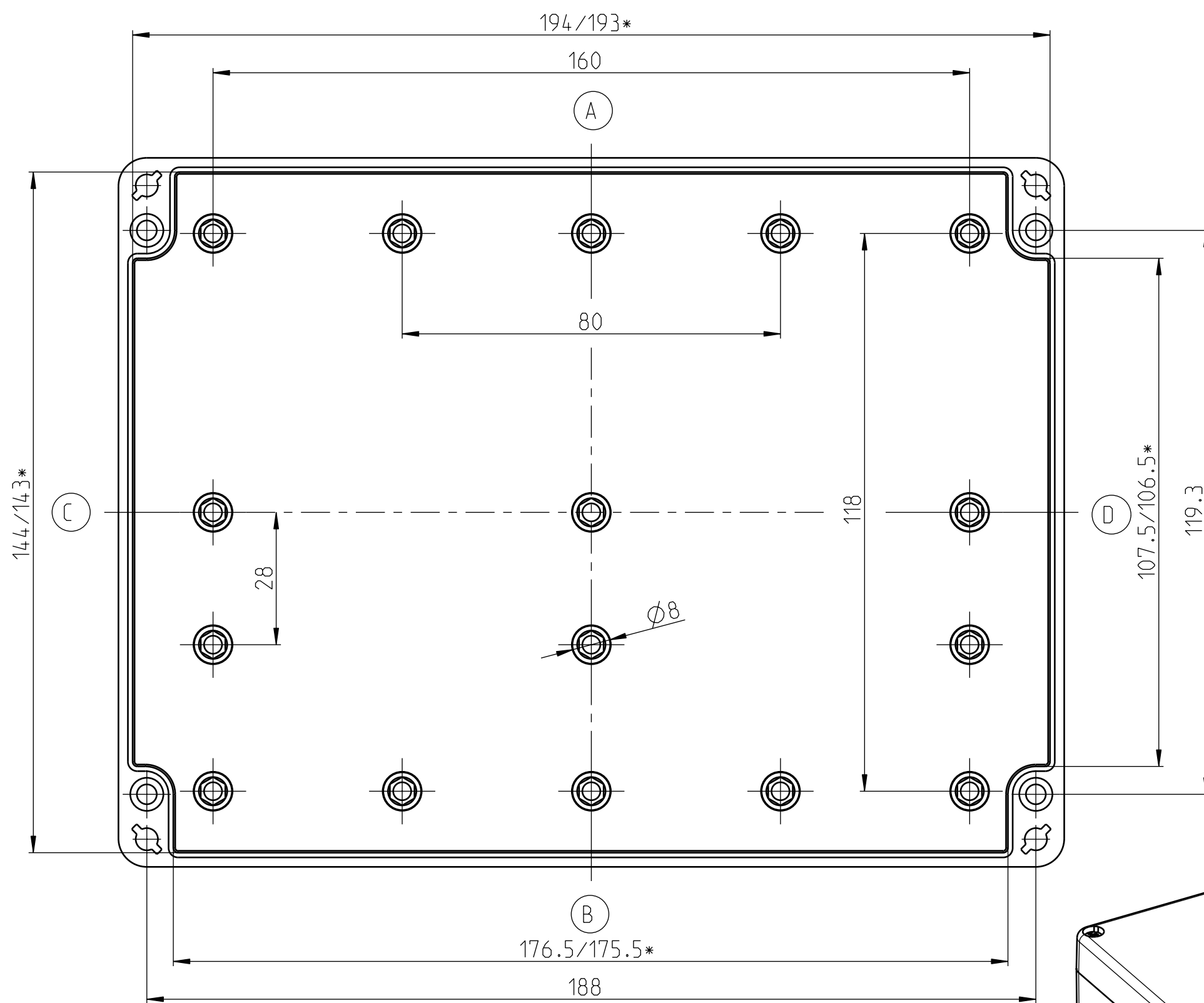
UNTERTEIL/BASE/PARTIE BASSE
