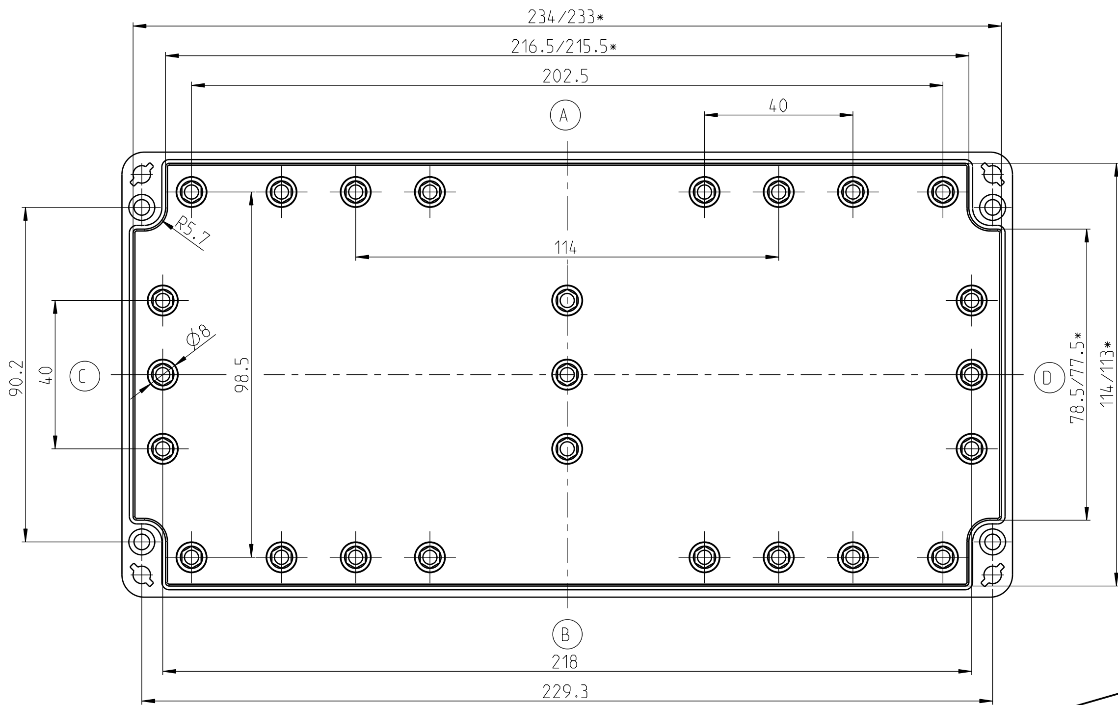
UNTERTEIL/BASE/PARTIE BASSE
