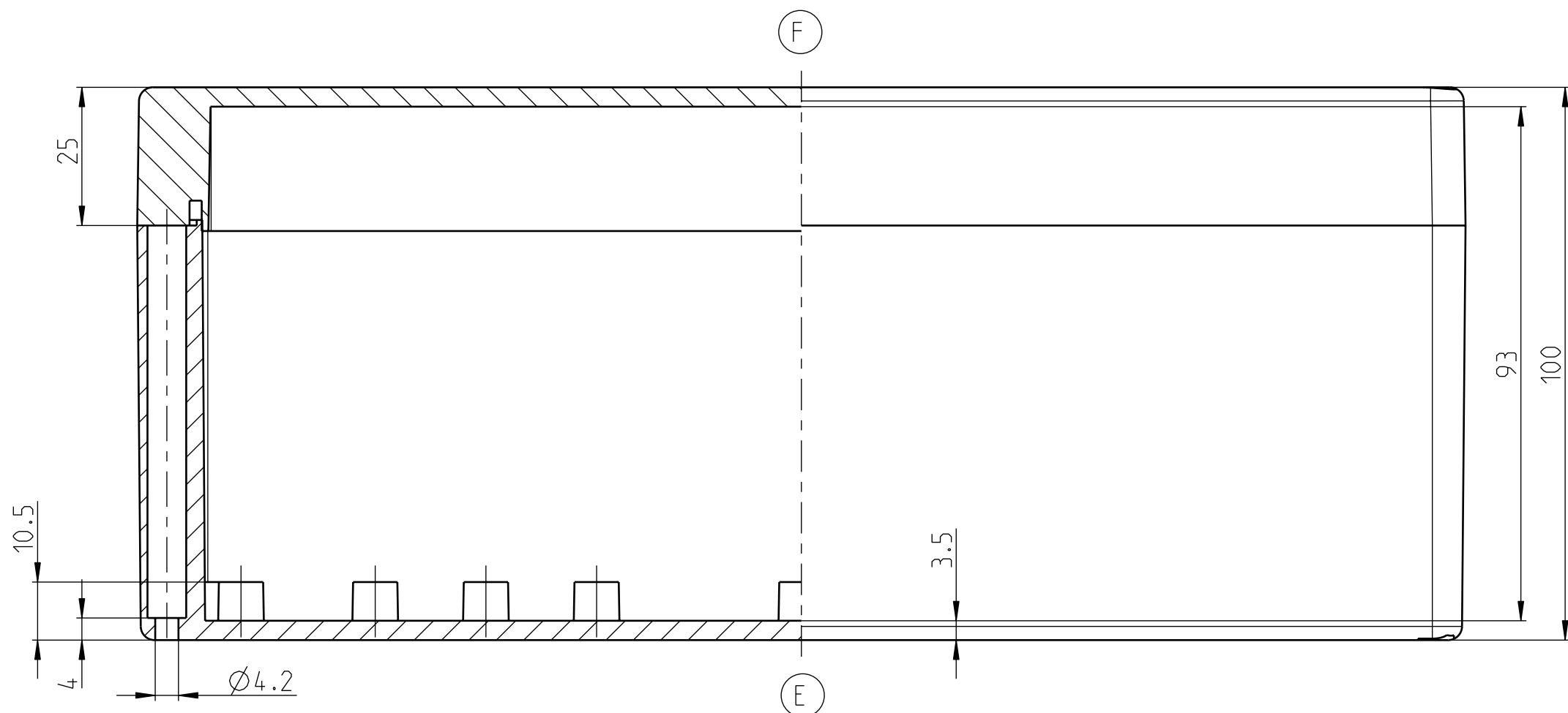
UNTERTEIL/BASE/PARTIE BASSE
