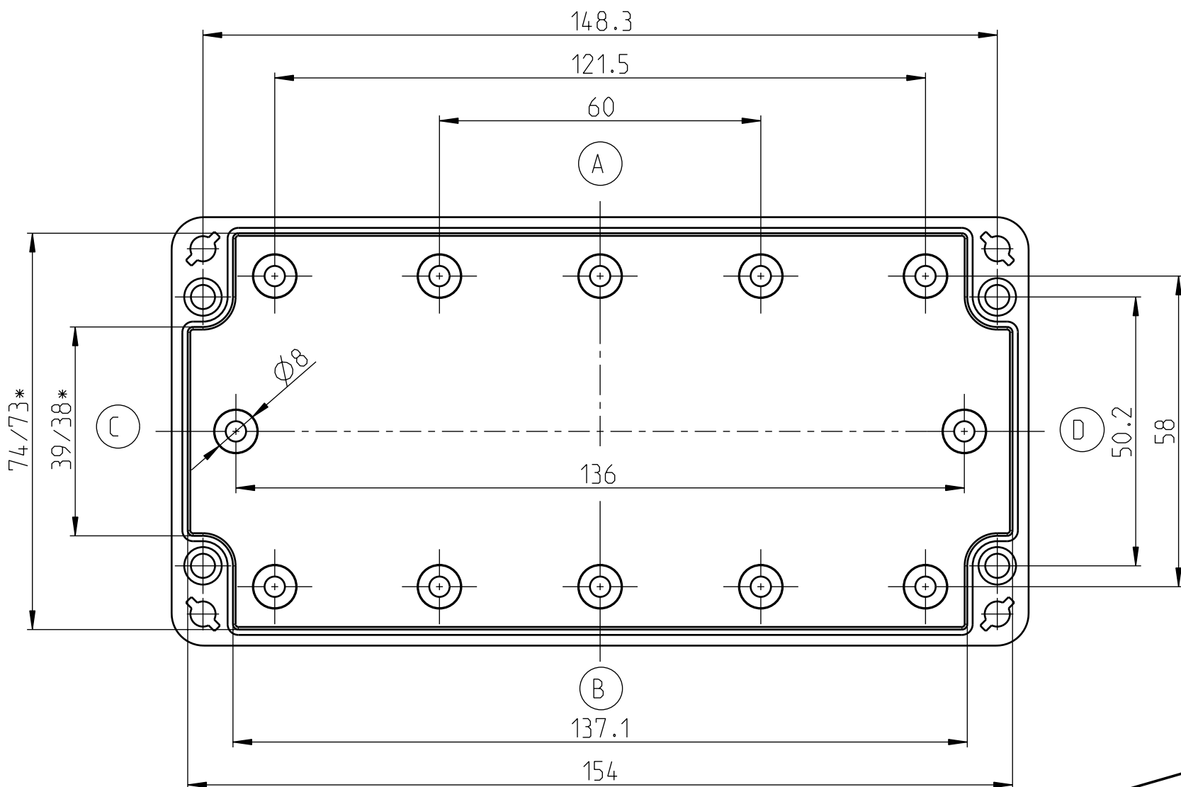
UNTERTEIL/BASE/PARTIE BASSE
