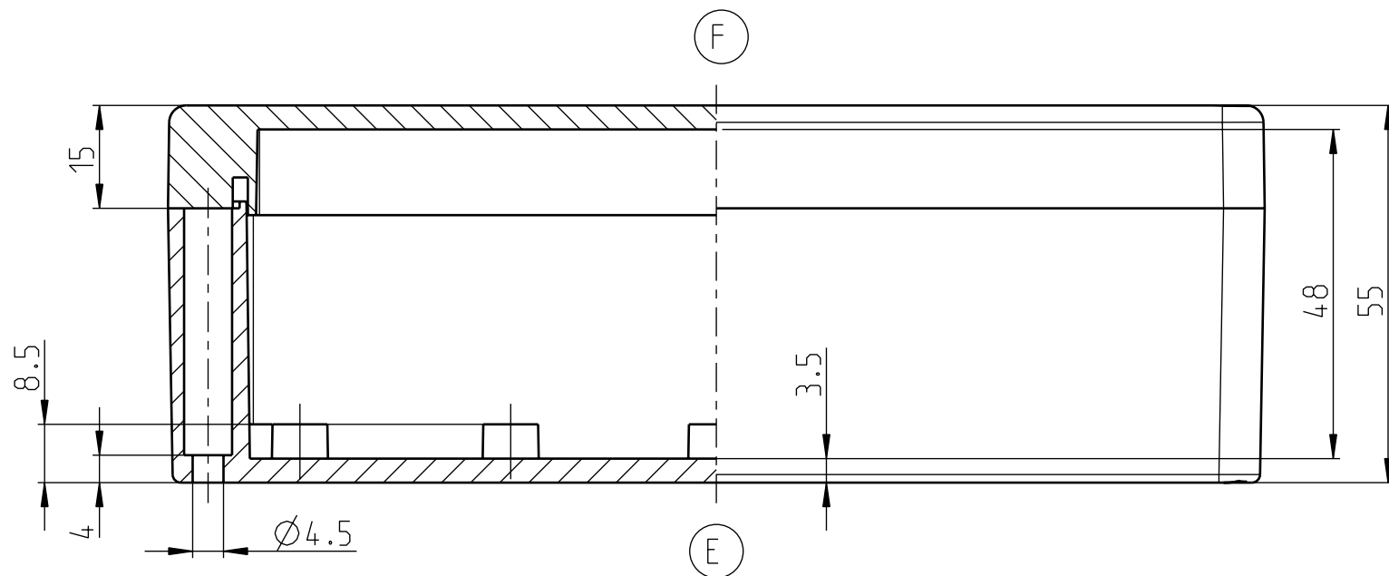
UNTERTEIL/BASE/PARTIE BASSE
