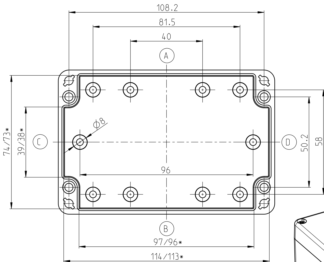
UNTERTEIL/BASE/PARTIE BASSE
