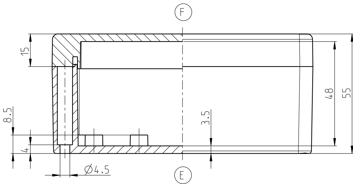
UNTERTEIL/BASE/PARTIE BASSE
