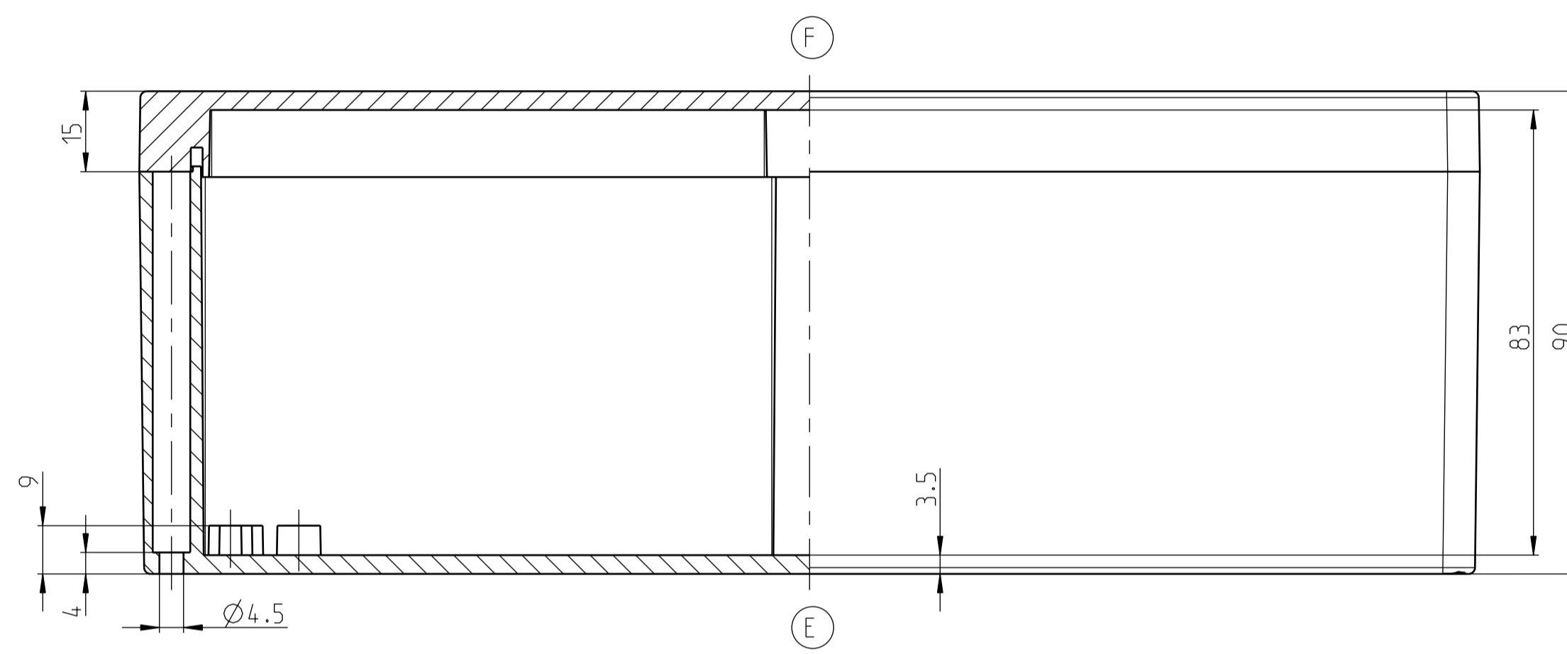
UNTERTEIL/BASE/PARTIE BASSE
