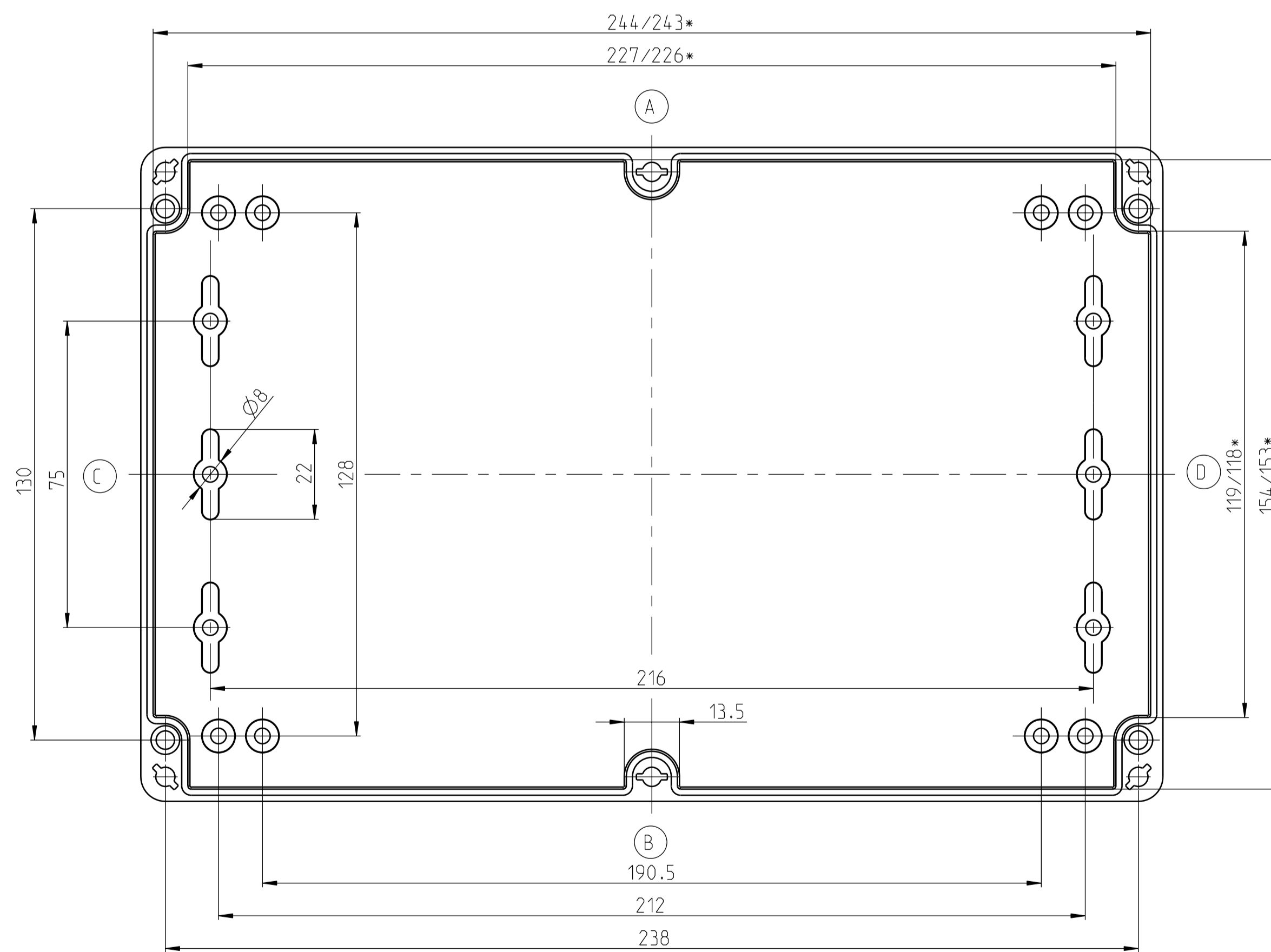
UNTERTEIL/BASE/PARTIE BASSE
