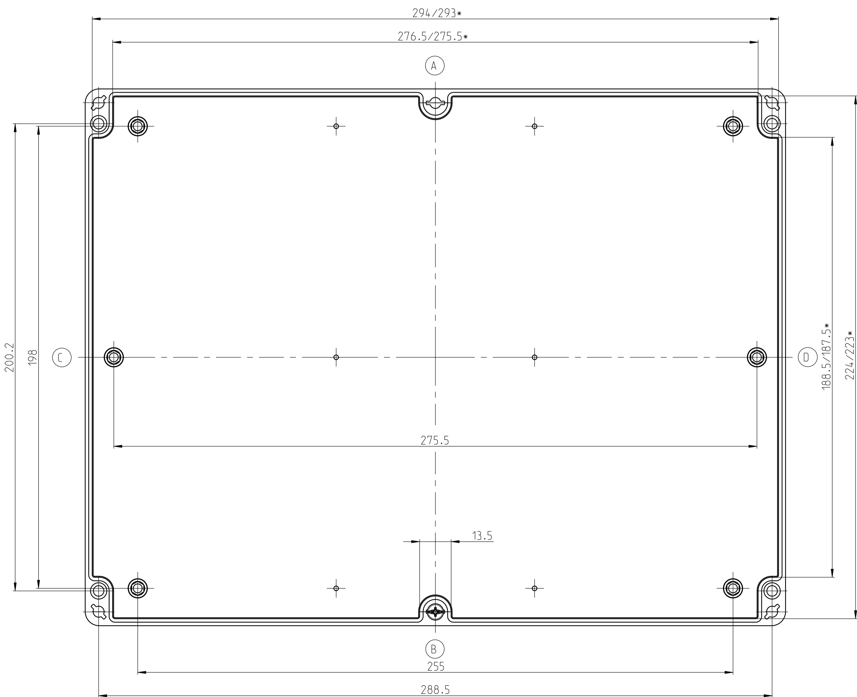
UNTERTEIL/BASE/PARTIE BASSE
