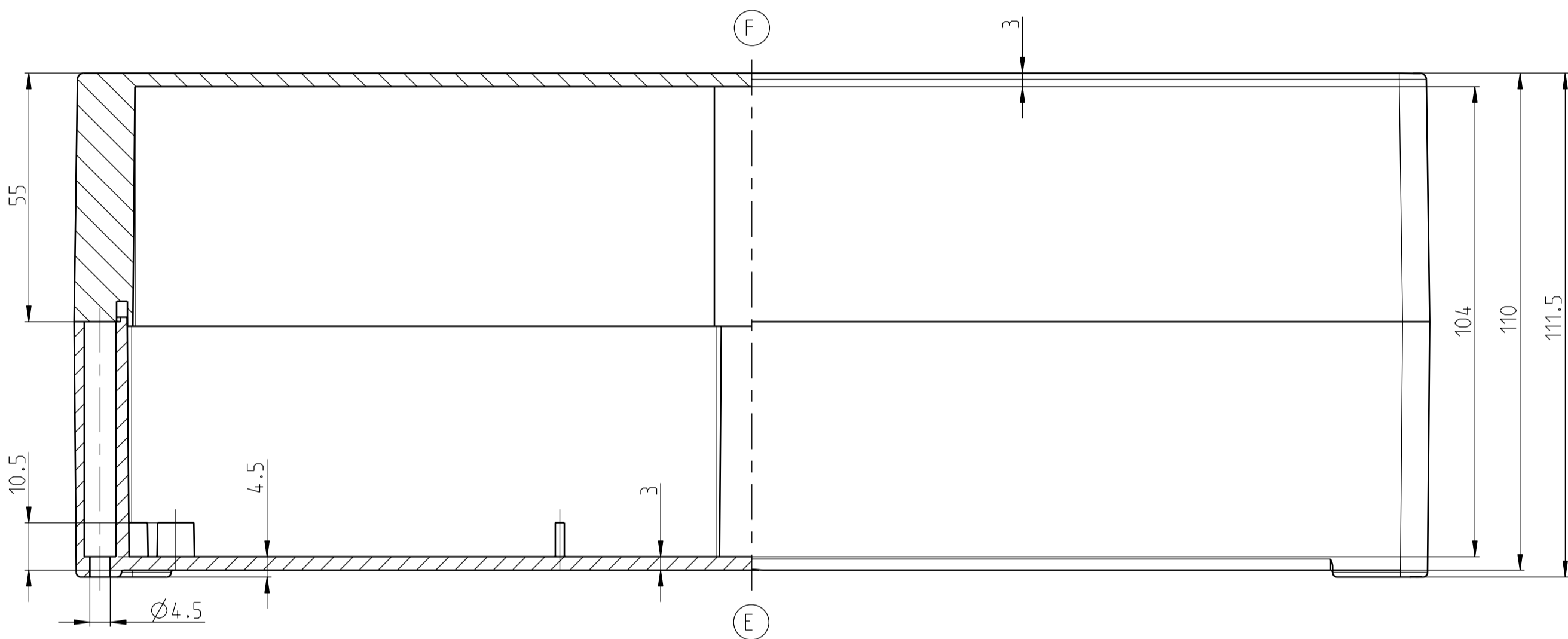
UNTERTEIL/BASE/PARTIE BASSE
