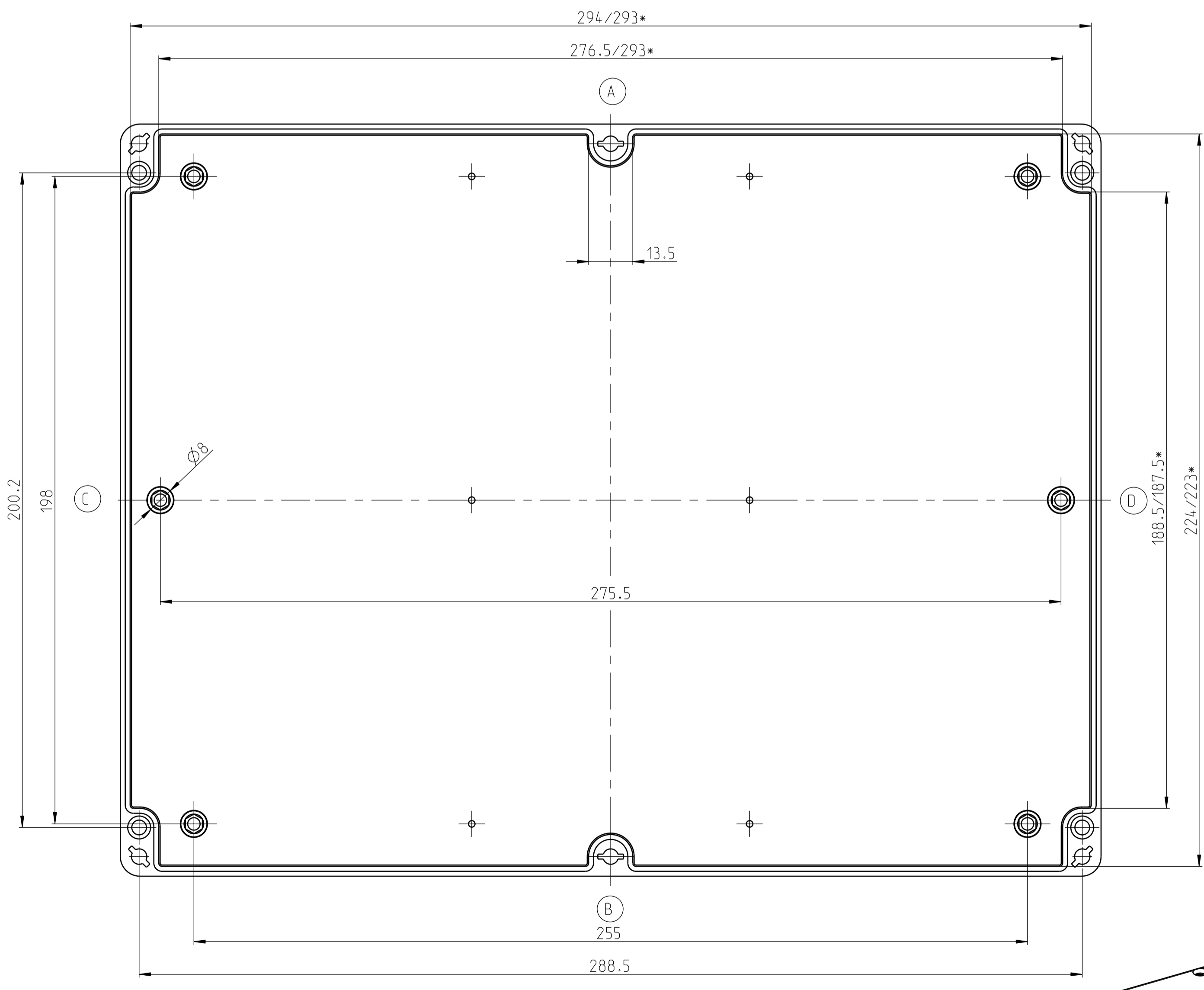
UNTERTEIL/BASE/PARTIE BASSE
