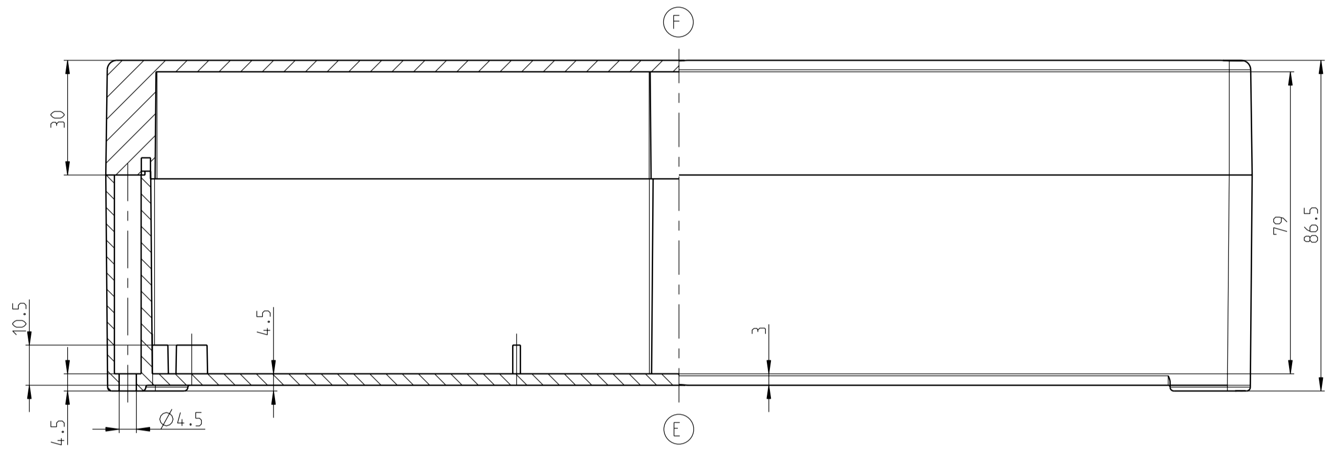
UNTERTEIL/BASE/PARTIE BASSE
