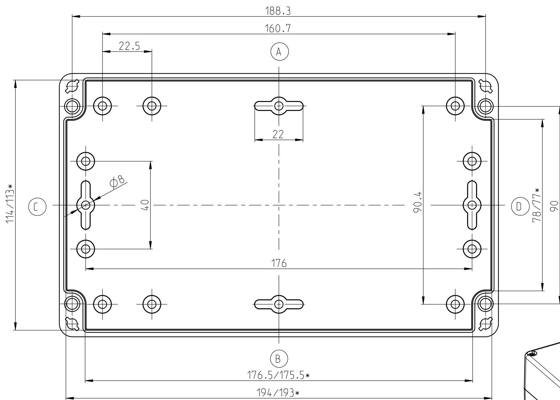
UNTERTEIL/BASE/PARTIE BASSE
