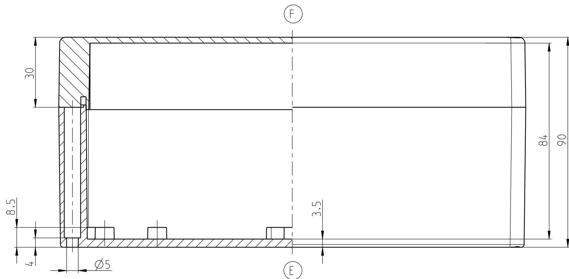
UNTERTEIL/BASE/PARTIE BASSE
