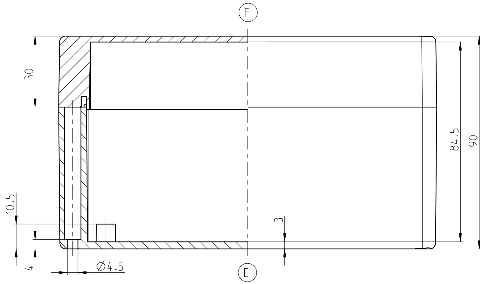
UNTERTEIL/BASE/PARTIE BASSE
