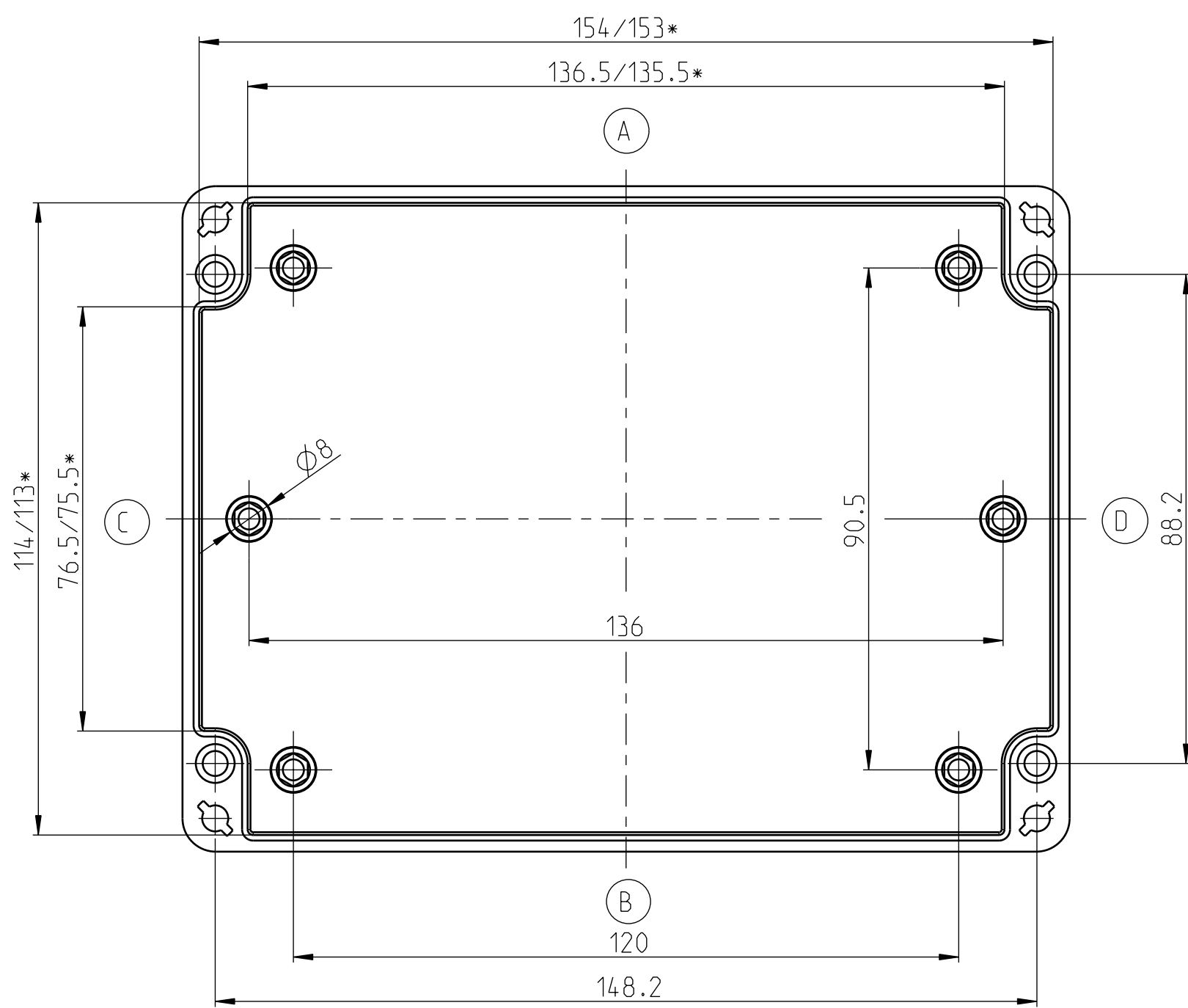
UNTERTEIL/BASE/PARTIE BASSE
