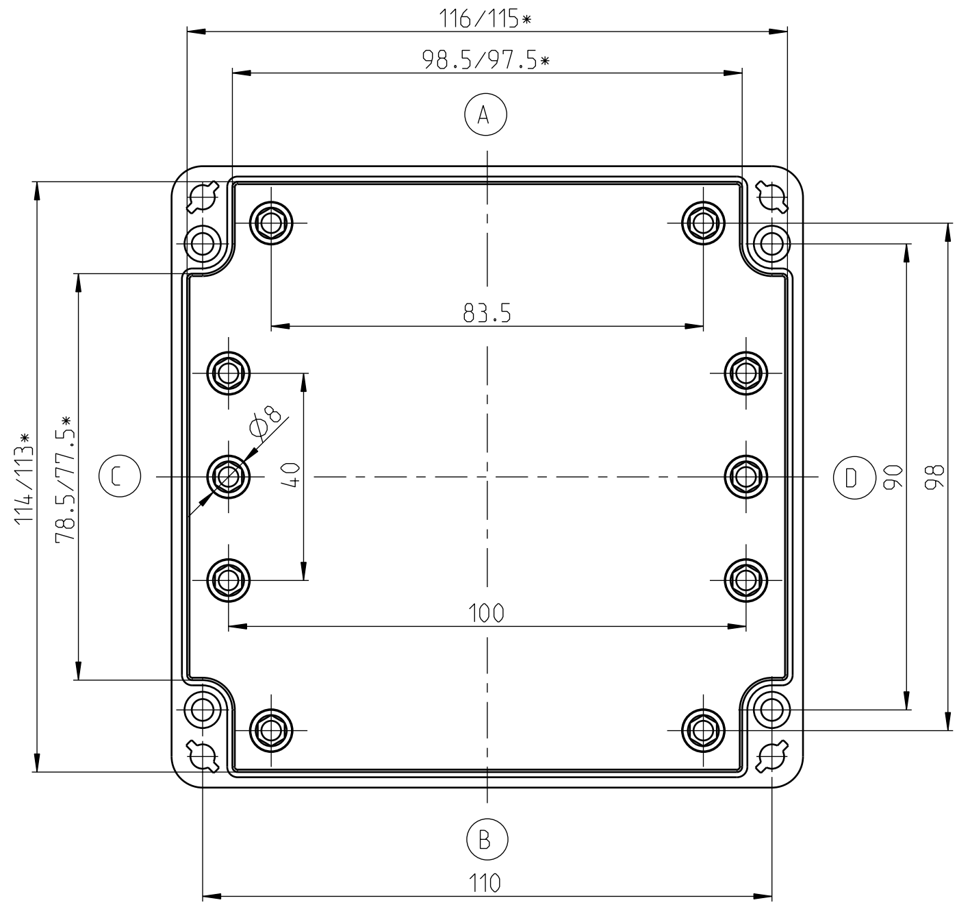
UNTERTEIL/BASE/PARTIE BASSE
