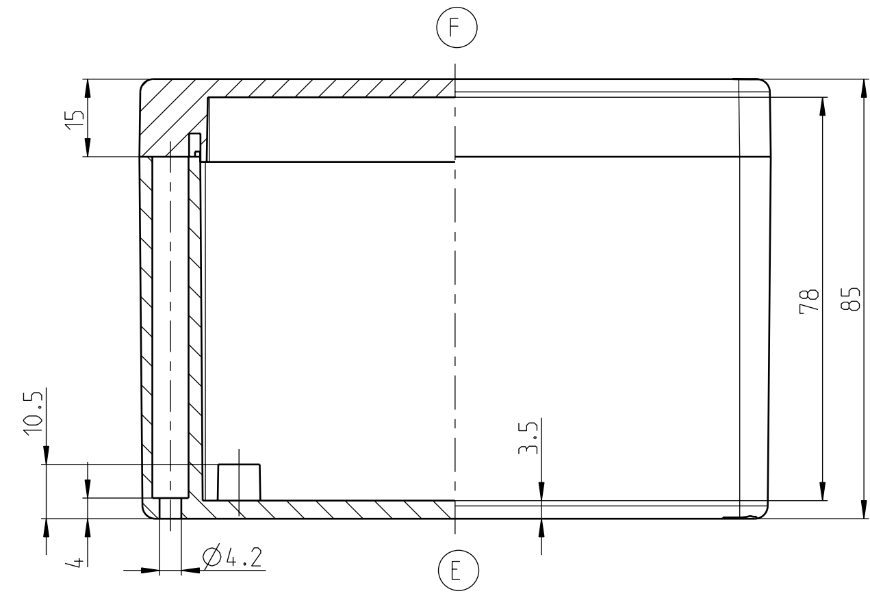
UNTERTEIL/BASE/PARTIE BASSE
