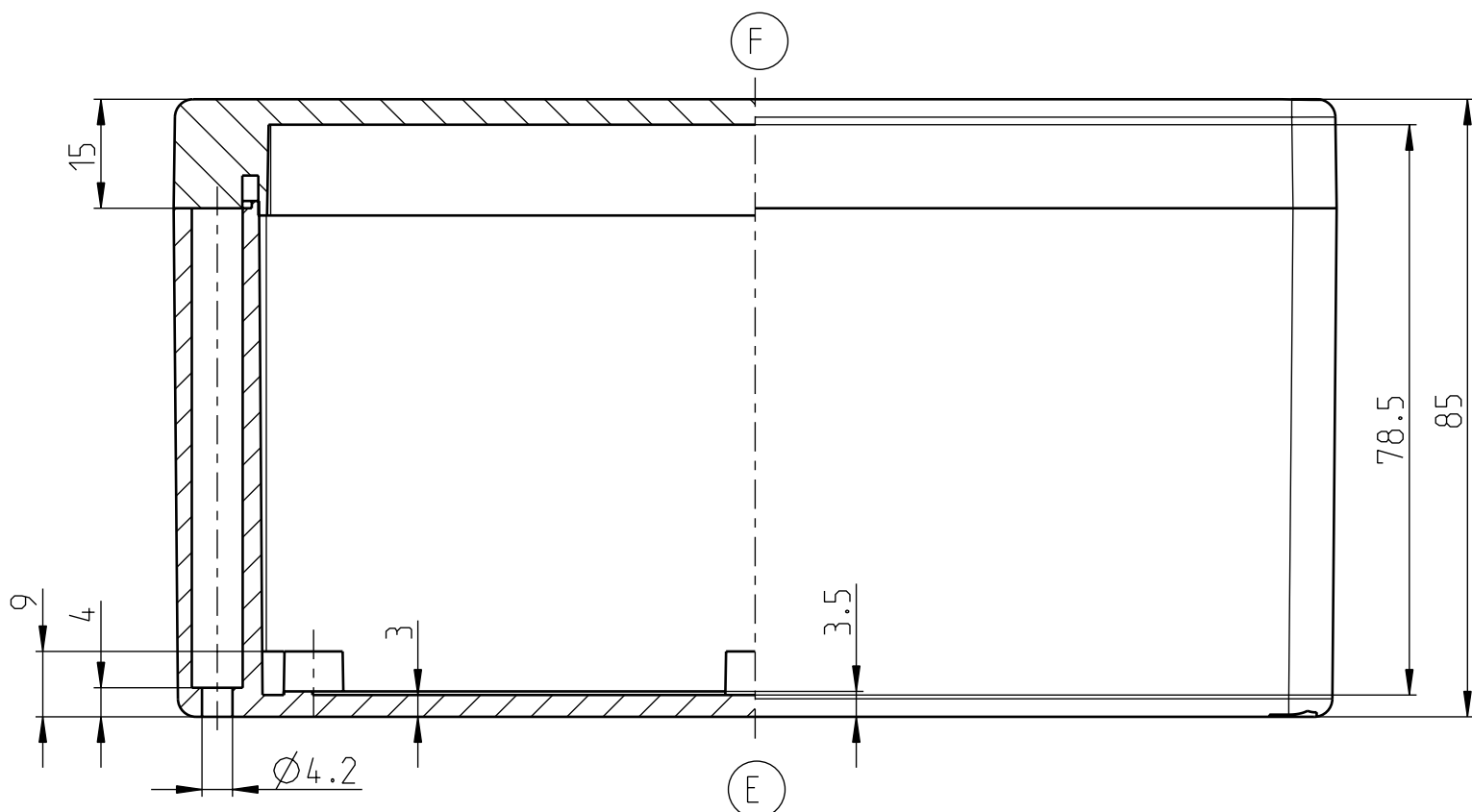
UNTERTEIL/BASE/PARTIE BASSE
