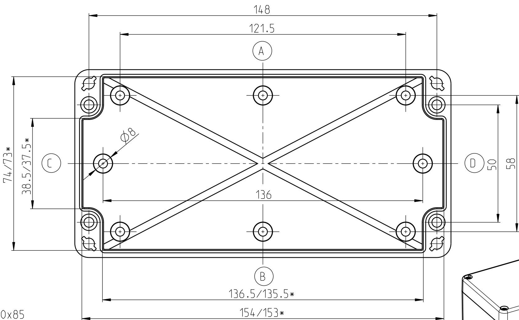
UNTERTEIL/BASE/PARTIE BASSE
