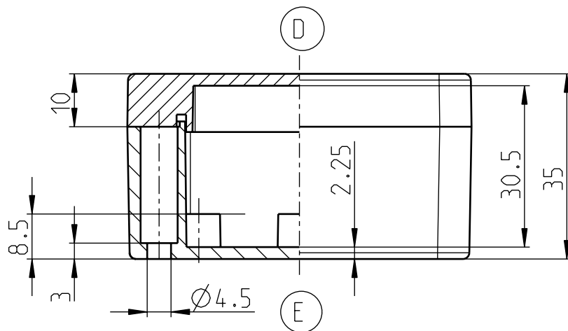
UNTERTEIL/BASE/PARTIE BASSE
