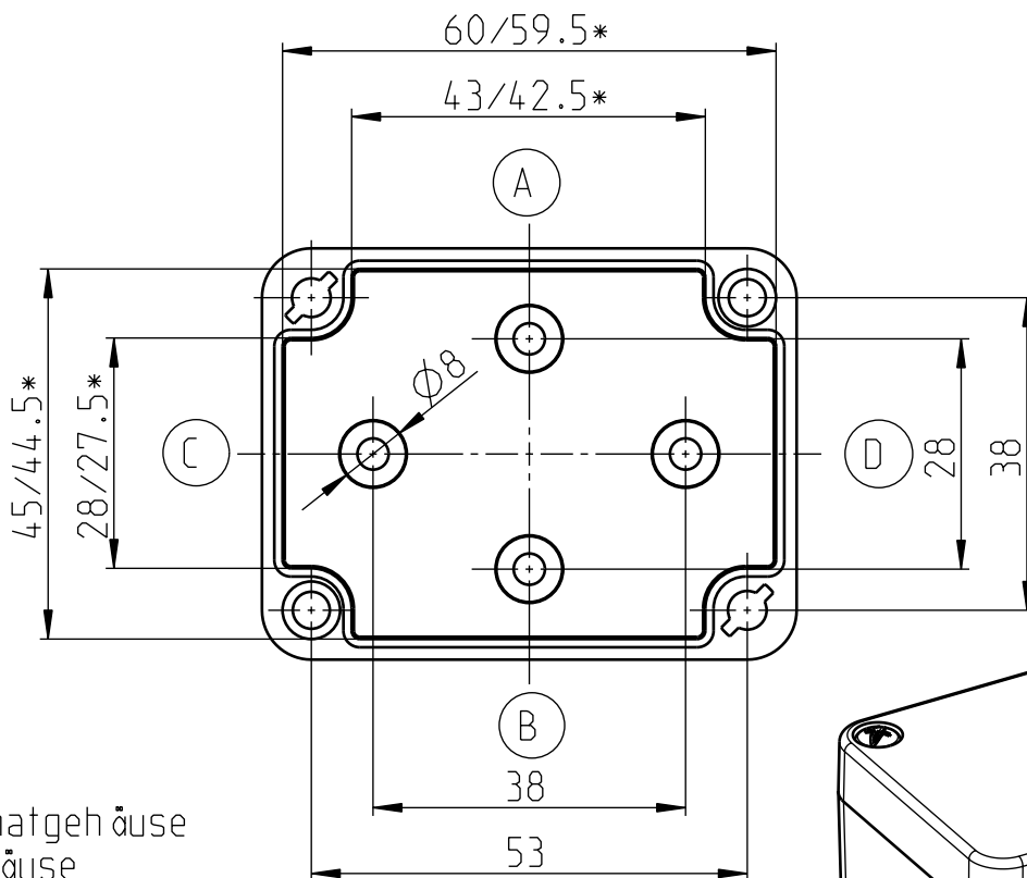
UNTERTEIL/BASE/PARTIE BASSE
