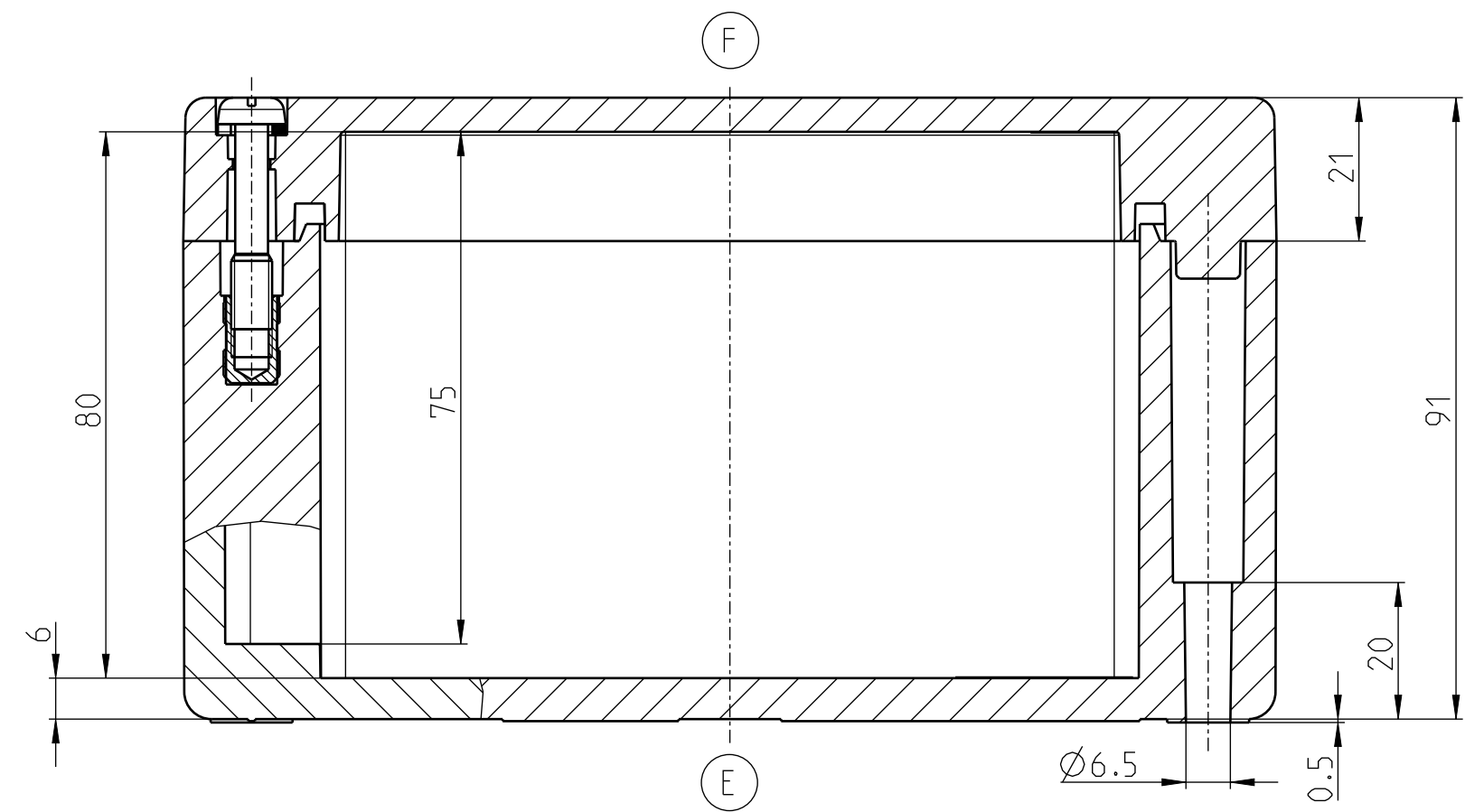
UNTERTEIL
