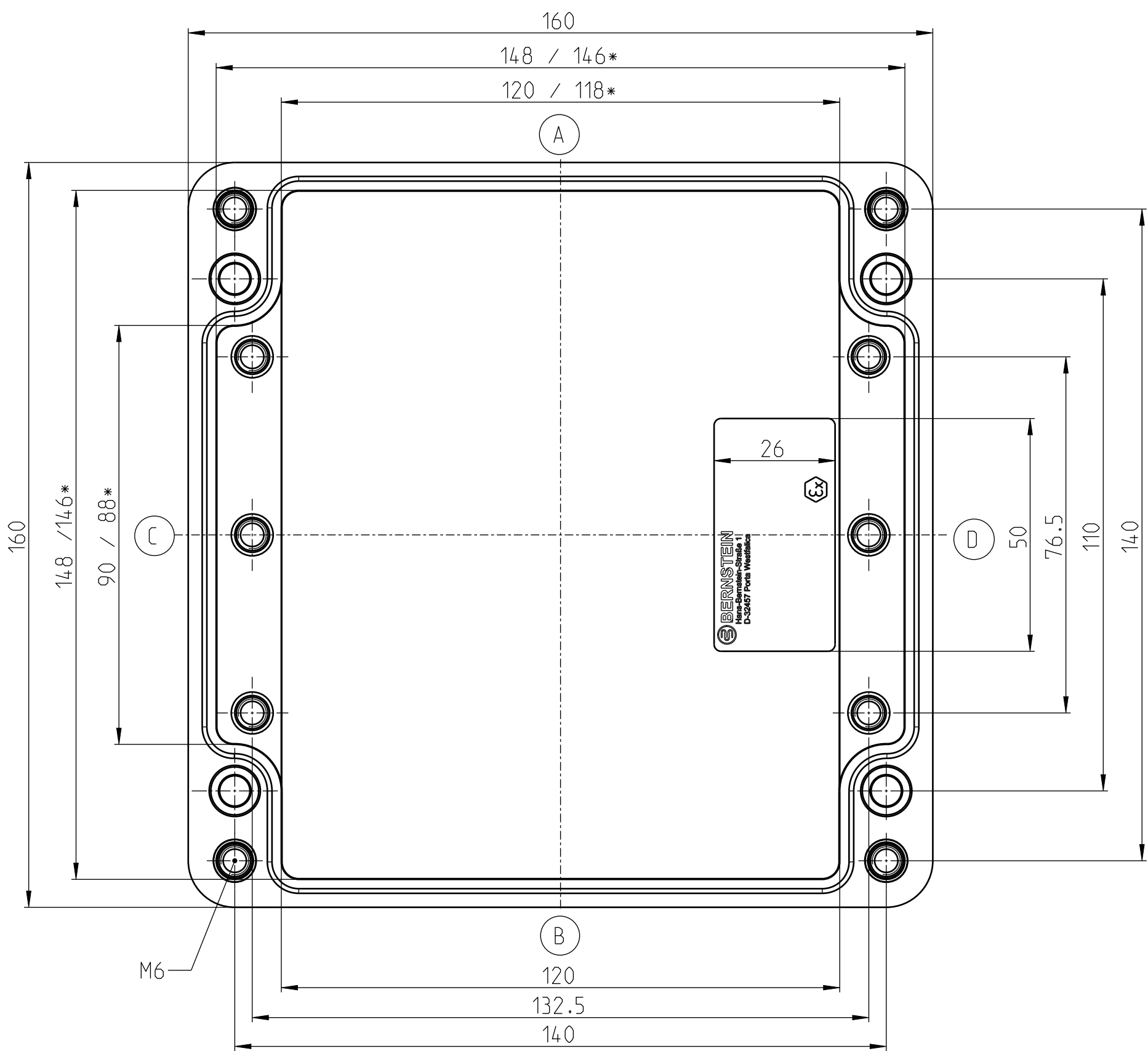
UNTERTEIL
