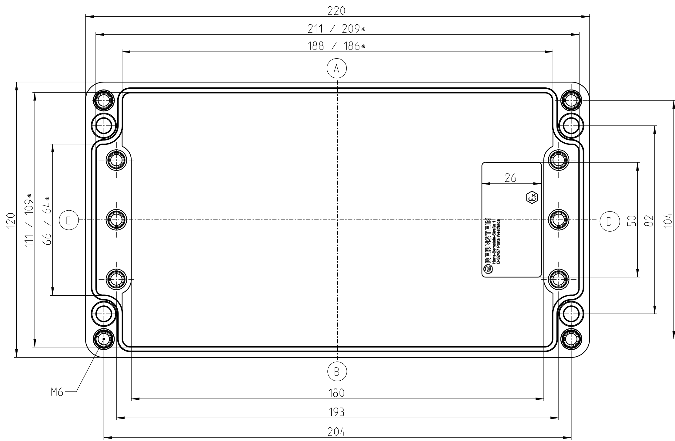
UNTERTEIL
