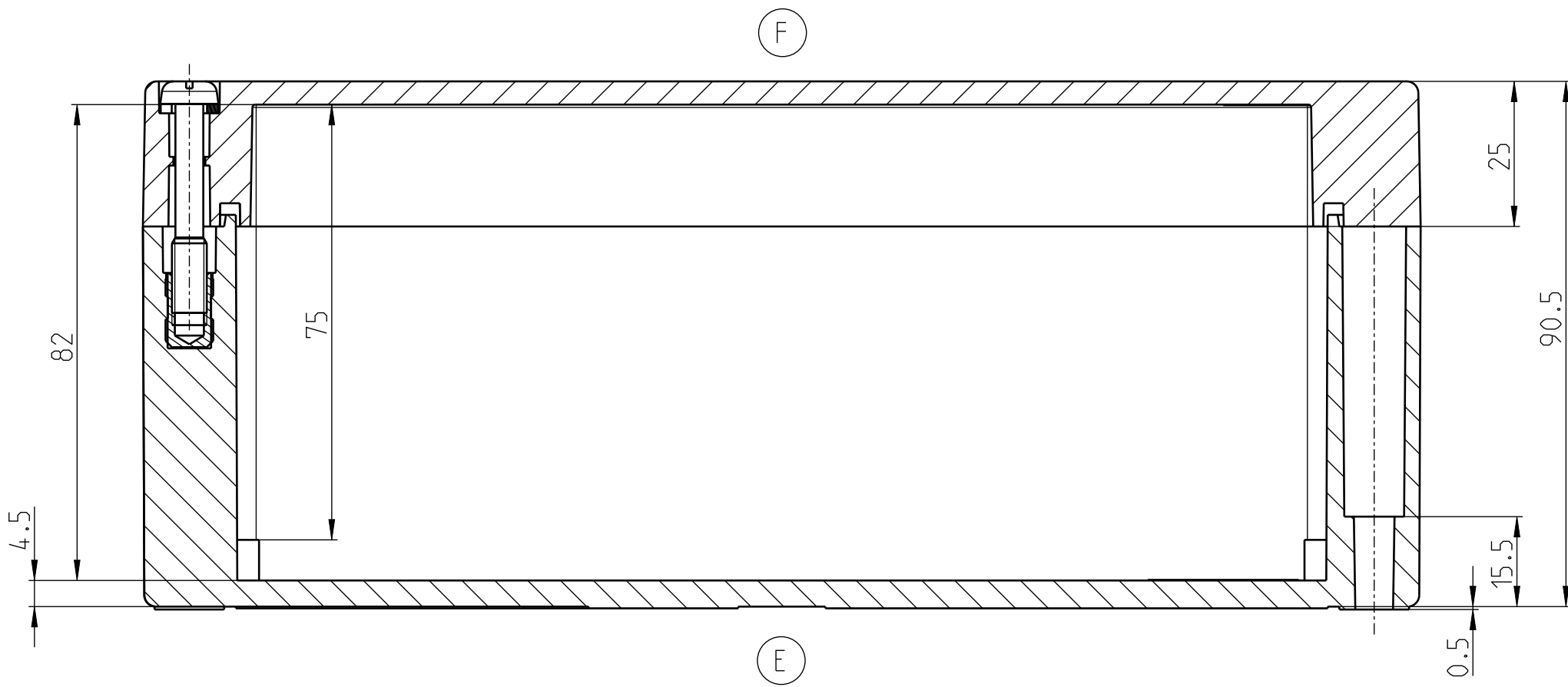
UNTERTEIL
