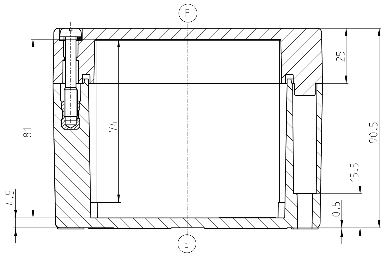
UNTERTEIL
