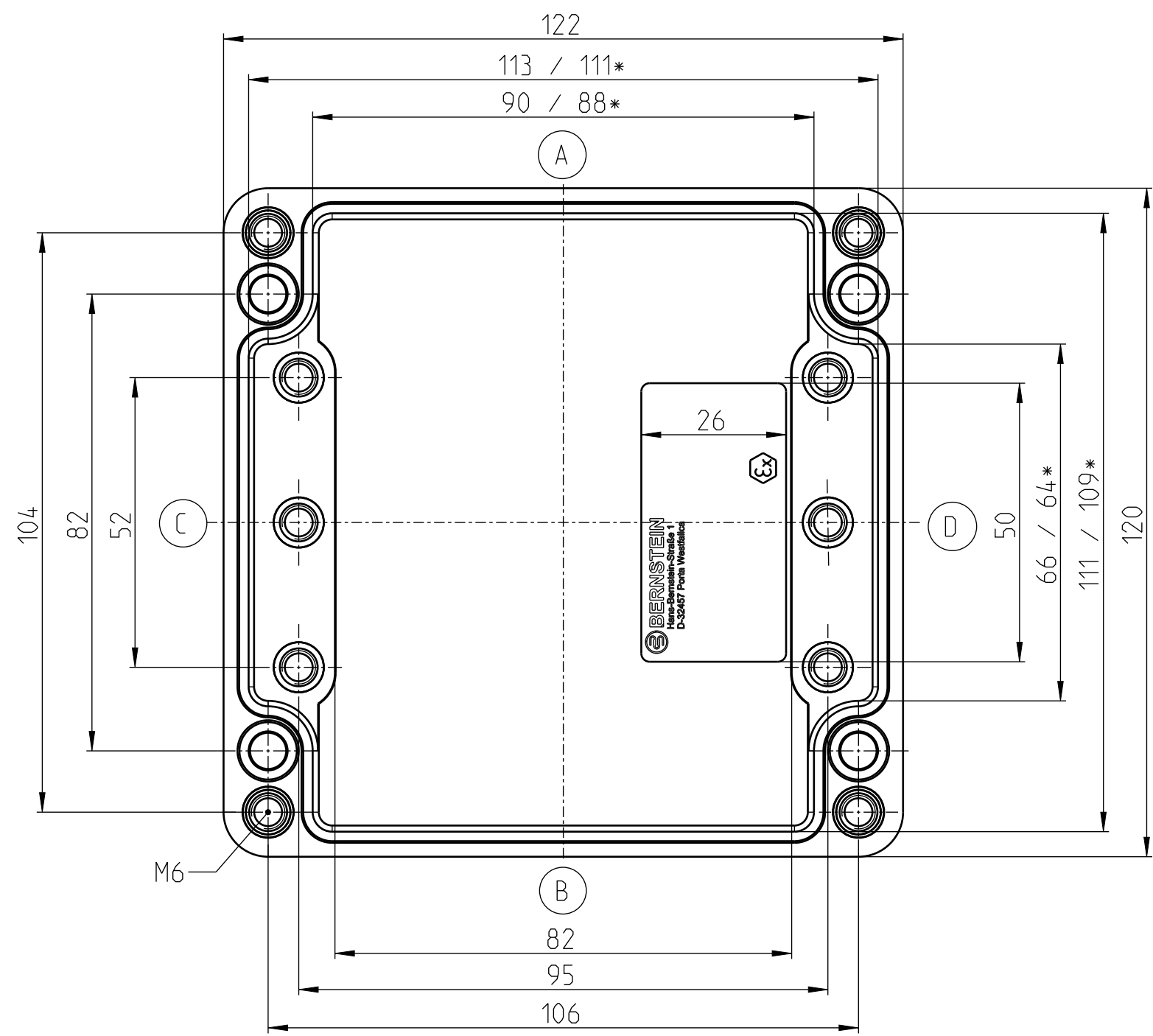
UNTERTEIL
