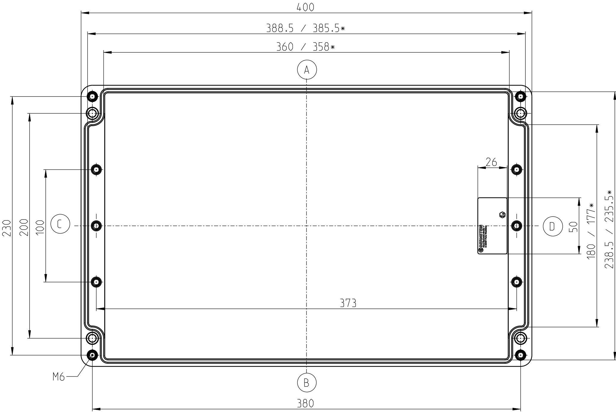
UNTERTEIL
