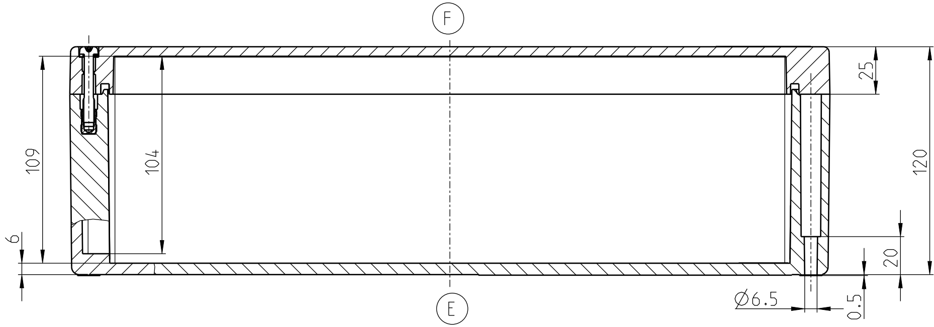
UNTERTEIL
