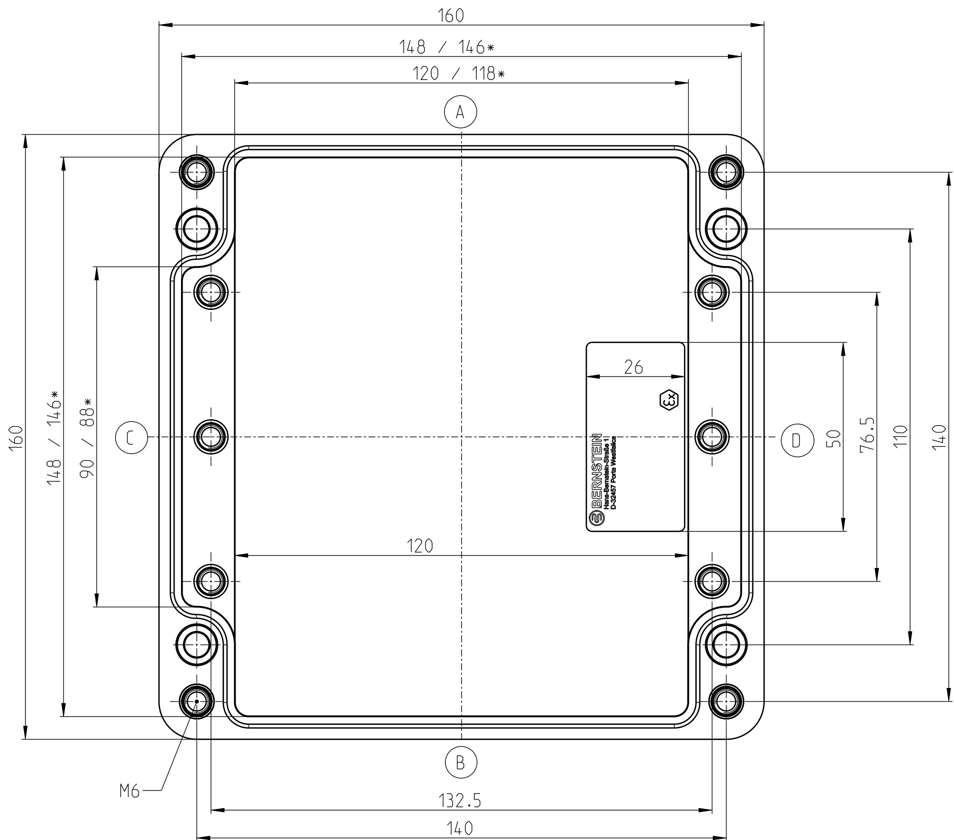
UNTERTEIL
