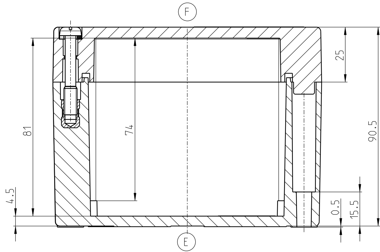
UNTERTEIL
