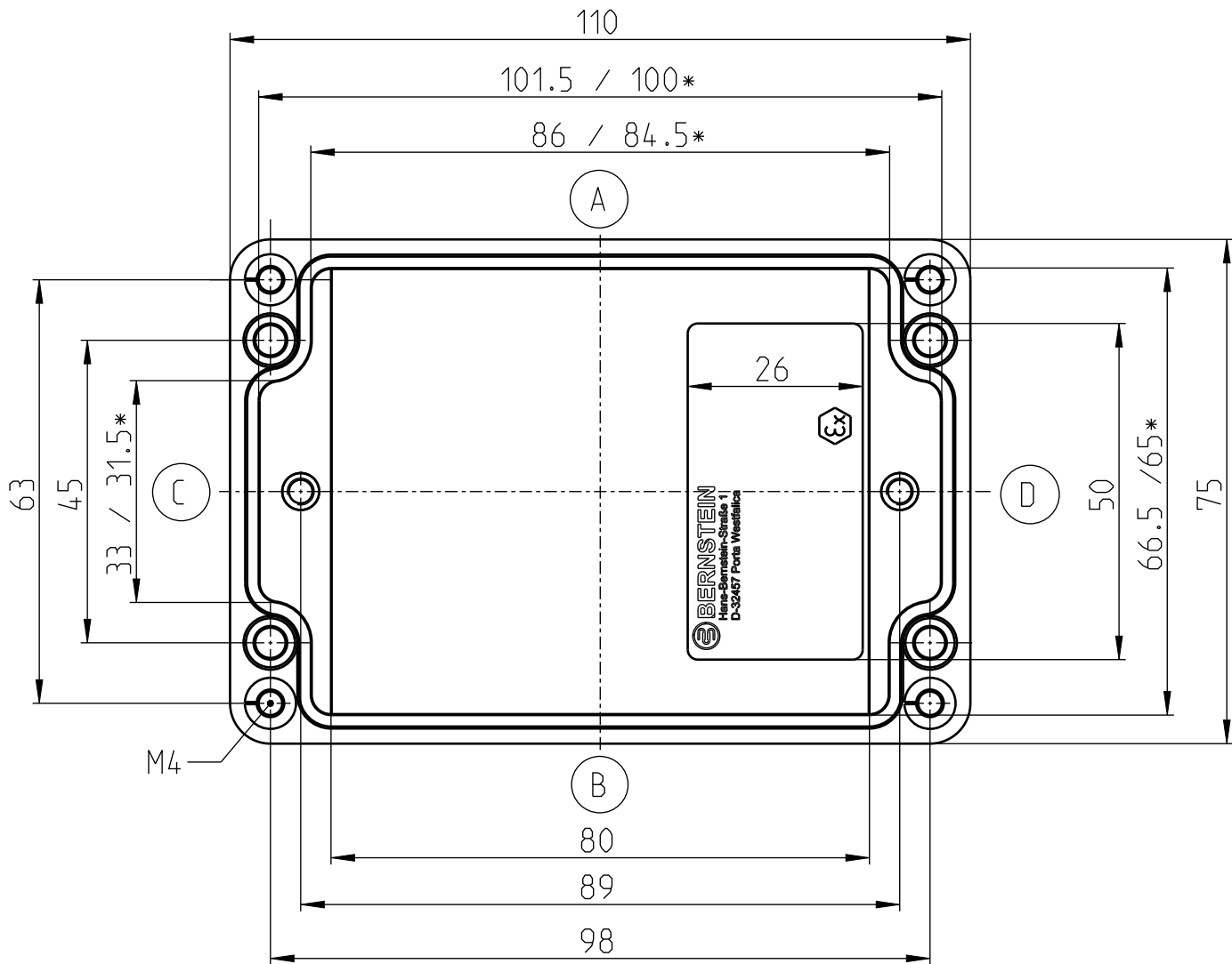
UNTERTEIL
