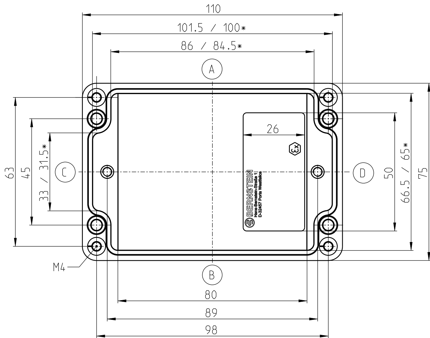
UNTERTEIL
