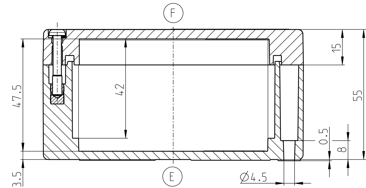
UNTERTEIL
