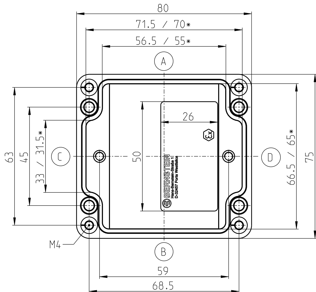
UNTERTEIL
